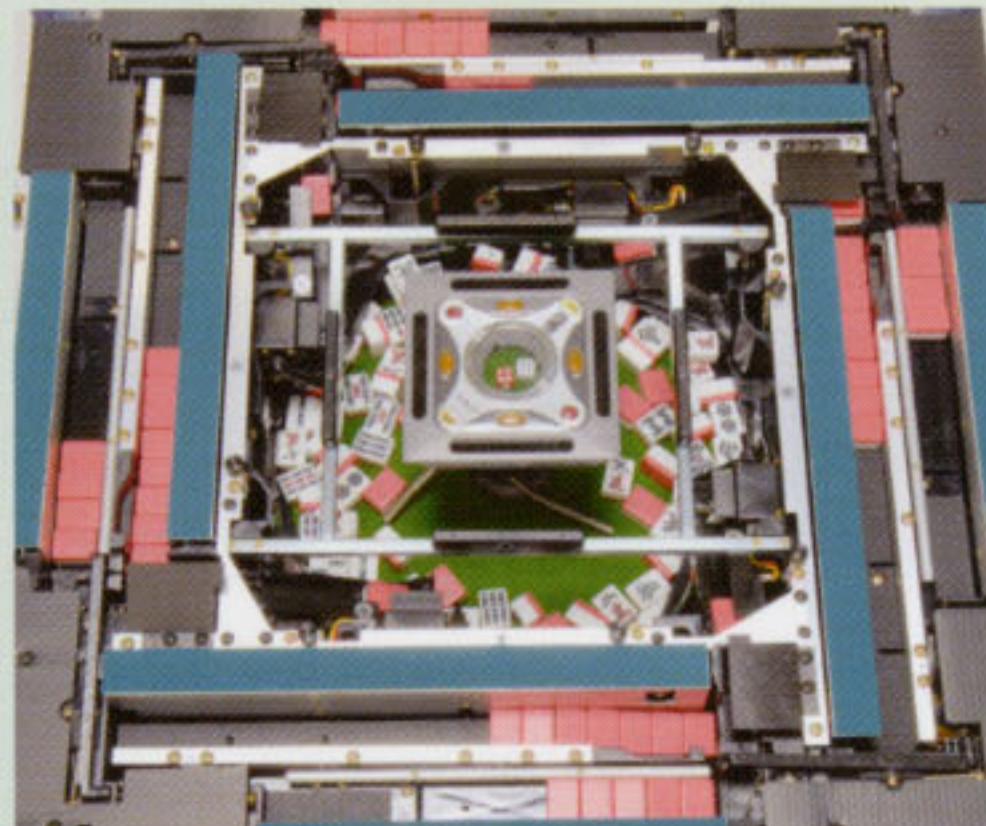
天板を開けた状態です。ホッパー内で牌が攪拌され、4カ所から同時に牌が吸い上げられます。
